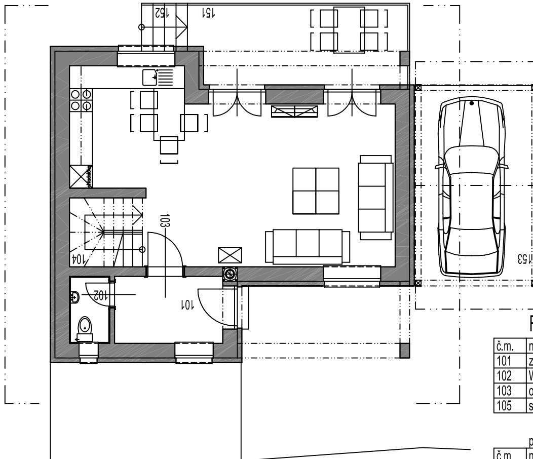
RD "B" - prízemie
